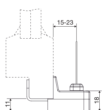
Seilbefestigung mit Klemmträger
